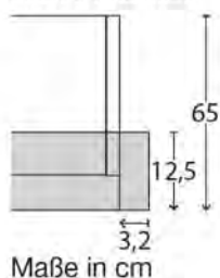
Draufsicht Schrank inkl. PPT-Rahmen
